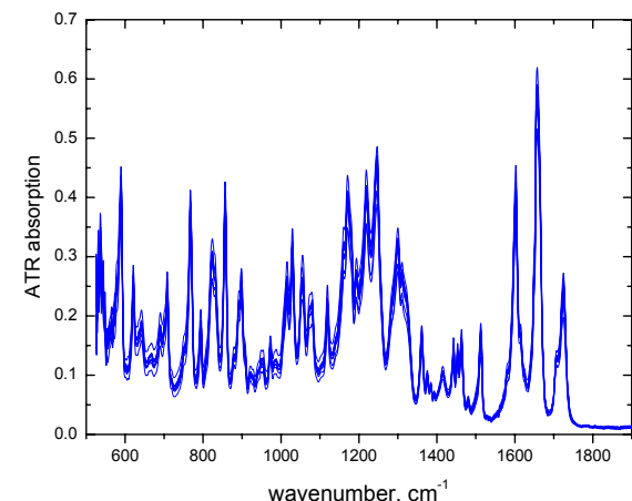
Σχήμα 2. Σύγκριση 11 διαφορετικών παρτίδων / περιεκτών φαρμακευτικής ουσίας μέσω των φασμάτων ATR. Τα φάσματα έχουν συλλεγεί με εξάρτημα διαμαντιού απλής ανάκλασης
